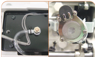
완전 자동 급유 시스템
