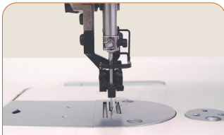
후물에 적합한 노루발 상승량
